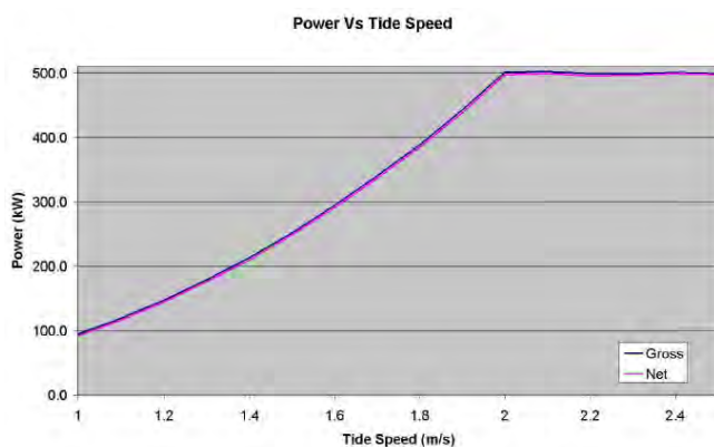
Figuur 12: Stingray “power curve” voor de geplande 2e generatie.
