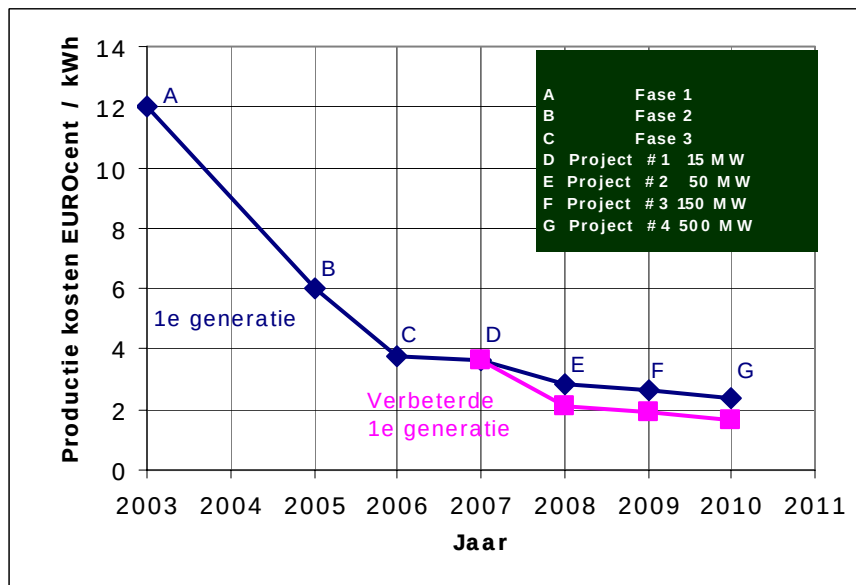
Figuur 8: Door MCT geprojecteerde elektriciteits productie kosten 1
